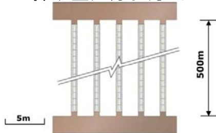
採鉱型処分孔方式
