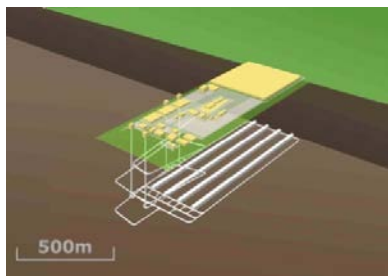
深孔処分方式
