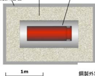
ベントナイト/ケイ砂混合 鋼製外容器 オーバーバック
