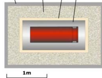
ベントナイト オーバーバック ケイ砂 鋼製外容器
